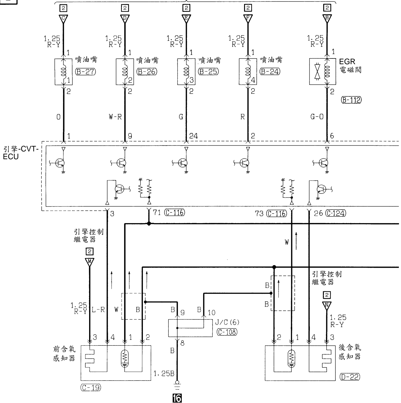
引擎控制幾電器
