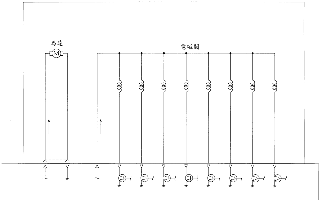
液壓單元
