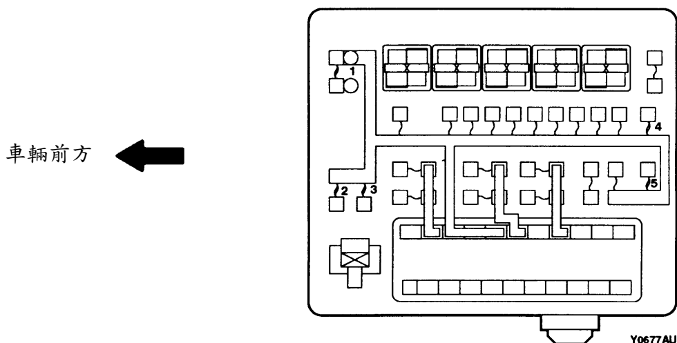
直接與電瓶正極連接之易熔絲
