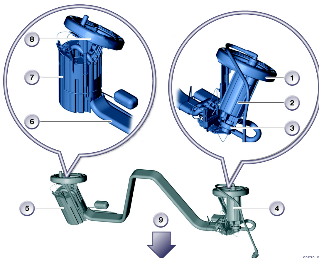
图 7: 燃油输送单元
