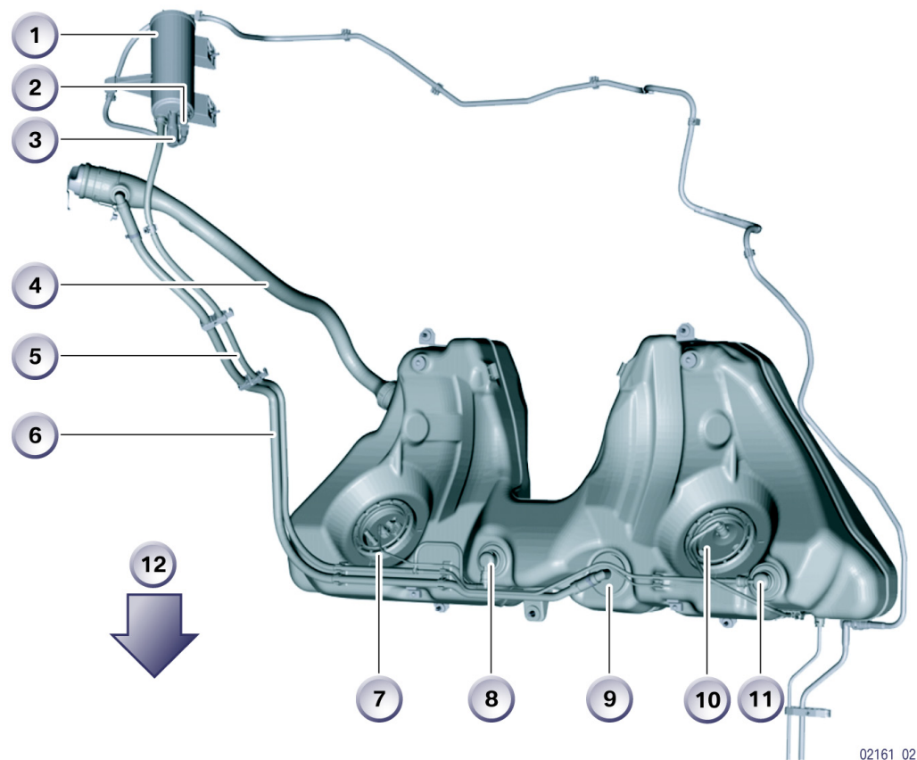
图 6: 燃油箱 (欧规, 汽油发动机)
