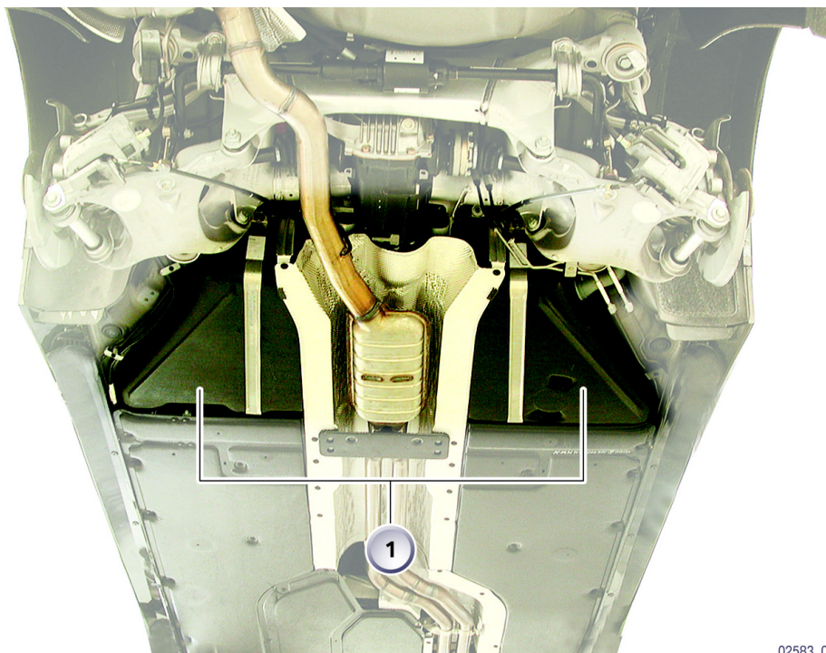
图 4: E60, 仰视图
