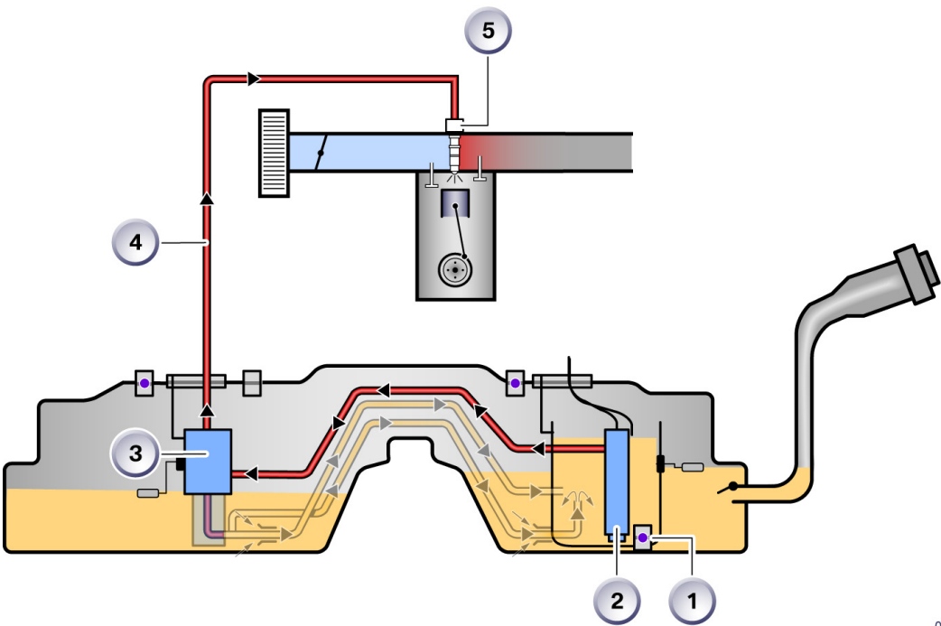
图 8: 燃油输送
