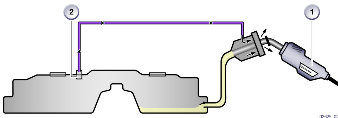
图 11: 加注管排气
