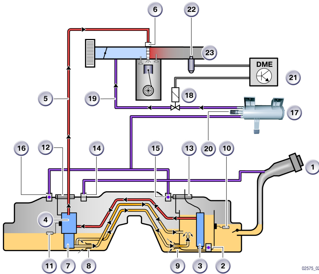
图 1: 燃油系统（欧规）
