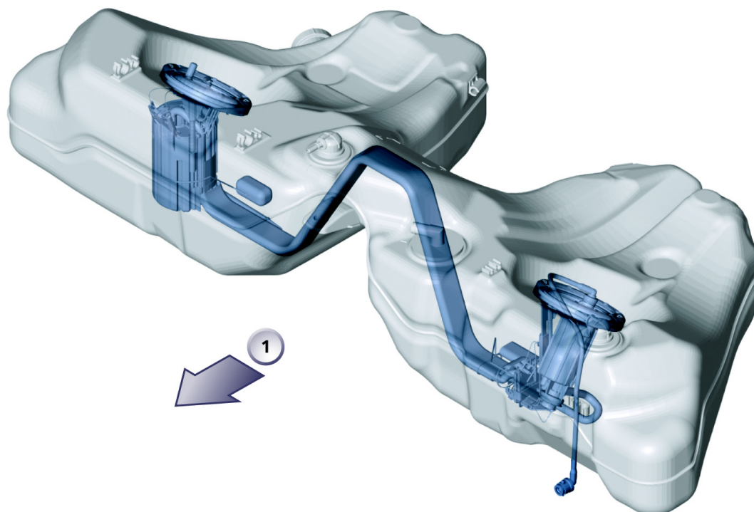
图 5: 燃油箱，行驶方向视图（1）
