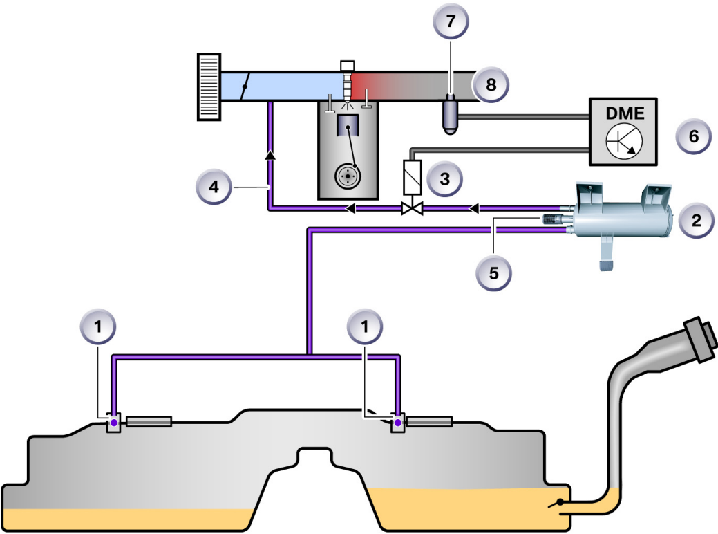
图 10: 运行排气
