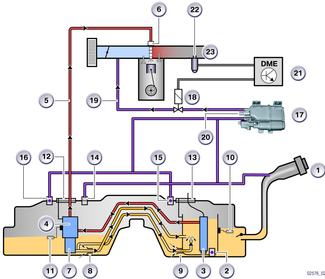
图 3: 燃油系统（美规，汽油发动机）
