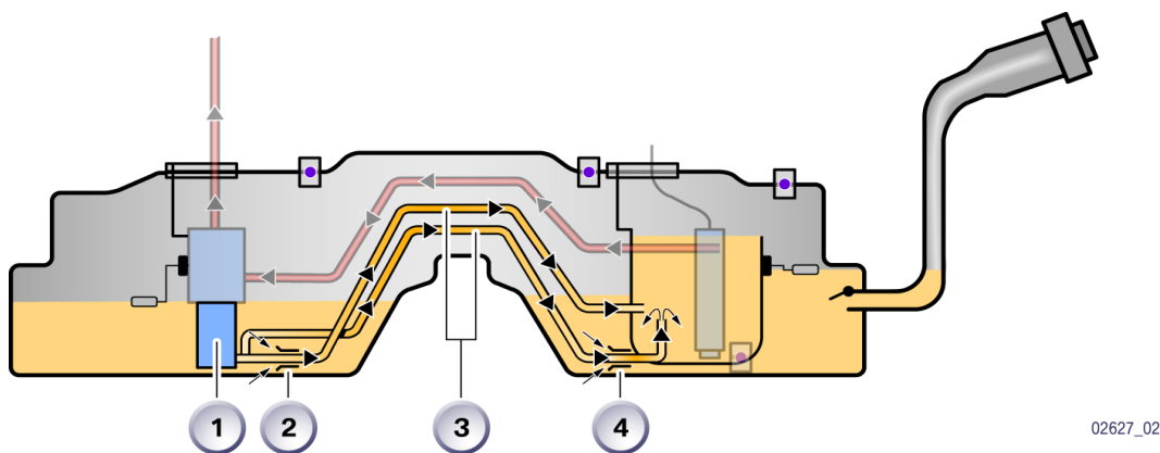
图 9: 燃油压力调节
