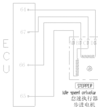
怠速执行器步进电机图
