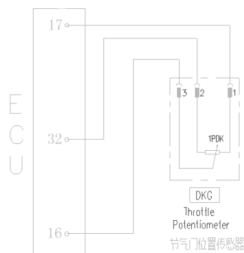
节气门位置传感器电路图
