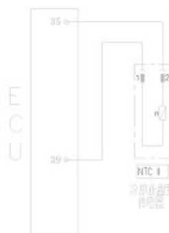
冷却液温度传感器电路图
