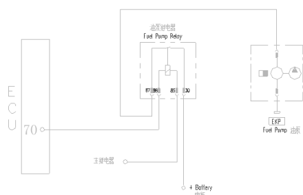
电动燃油泵电路图
