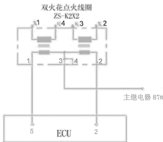
点火线圈电路图
