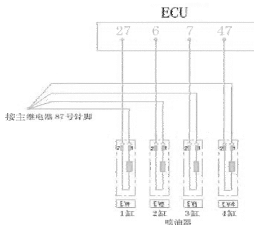
电磁喷油器电路图
