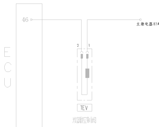
炭罐控制阀
