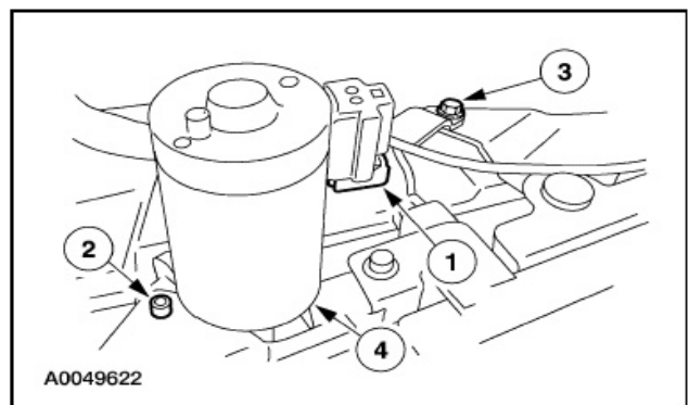
前高度电机
