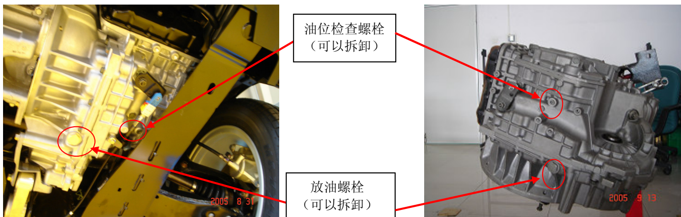
油位检查螺栓和放油螺栓位置示意图
