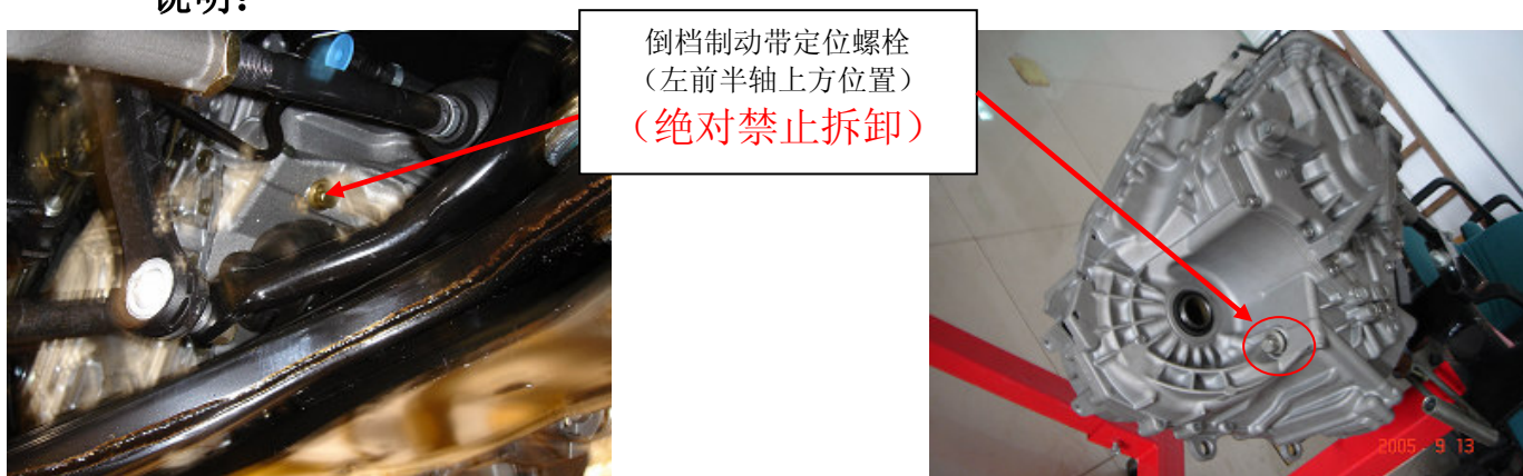
倒档制动带固定螺栓位置示意图
