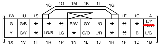
G1-01 A/C AMPLIFIER (I) 空调放大器 (I)
