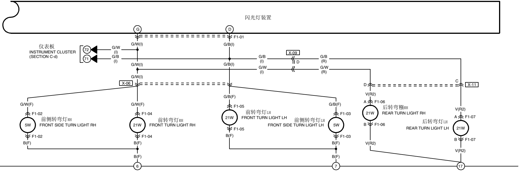
F1-01 FLASHER UNIT (I) 闪光灯装置
