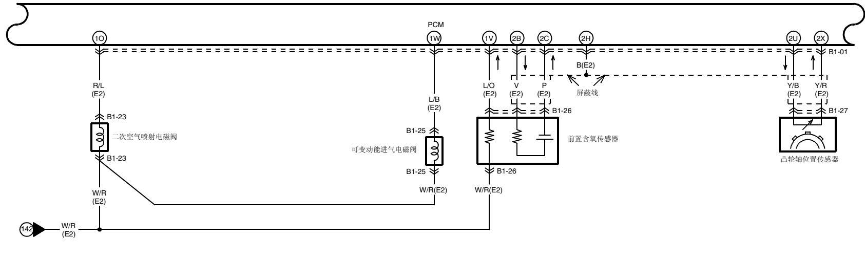
B1-23 二次空气喷射电磁阀 (E2)
