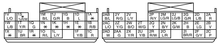
B1-25 可变的动进气电磁阀 (E2)
