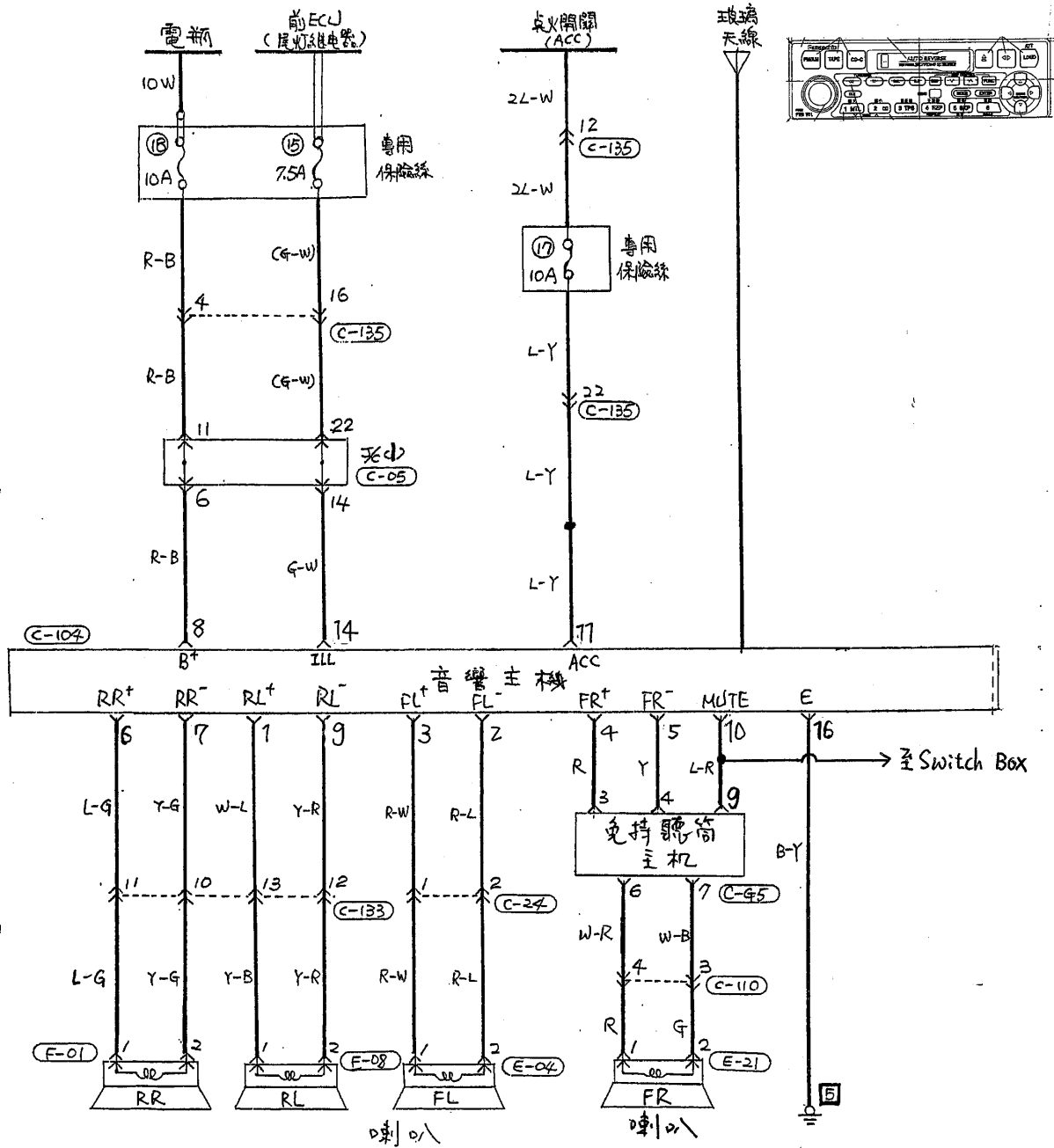
'03/05 <JT車> 迴路圖 — OSD 音响主机(藍芽)
