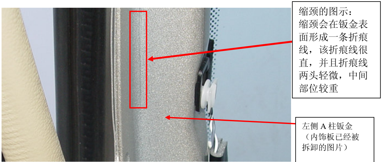
图二：左侧 A 柱钣金缩颈示意图
