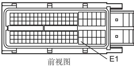
(C24) ECM 连接器
