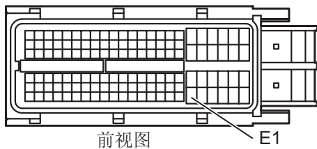
(C24) ECM 连接器
