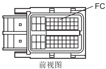
(A24) ECM 连接器
