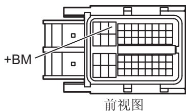
(A24) ECM 连接器
